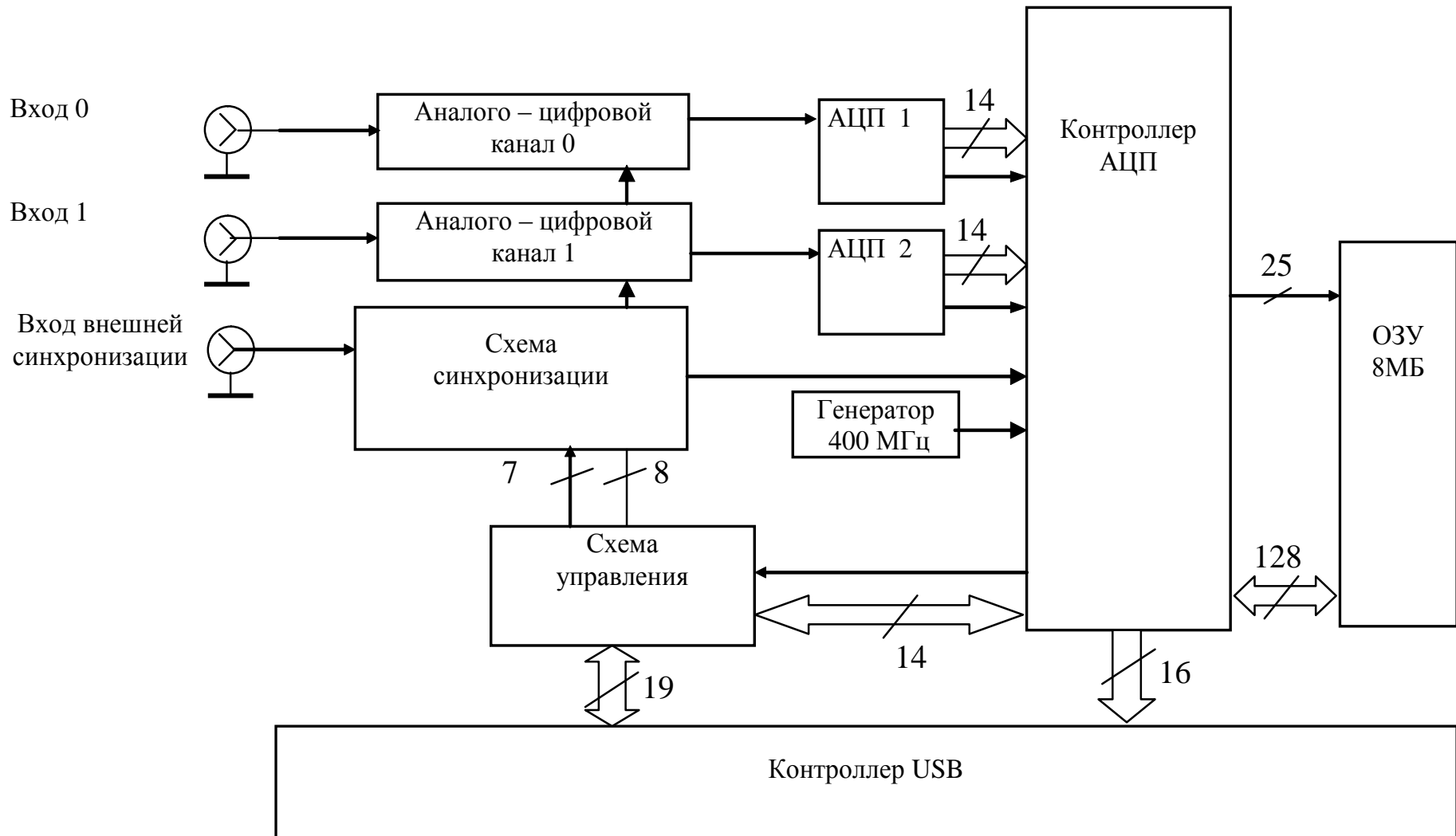
Рис. 5.1 Функциональная схема ЛА-n2USB-14
