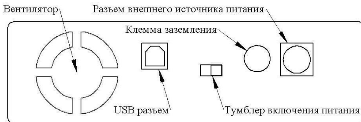
Рис. 4.1. Задняя панель прибора.
